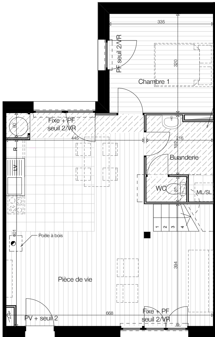
Plan de rez-de-chaussée
