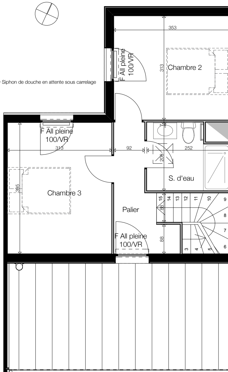
Plan de l'étage
